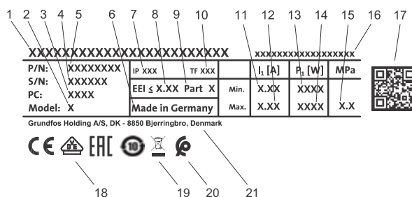
Abb. 19 Beispielhaftes Typenschild
