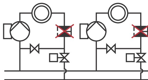
Abb. 27 Einsparen von Drosselventilen
