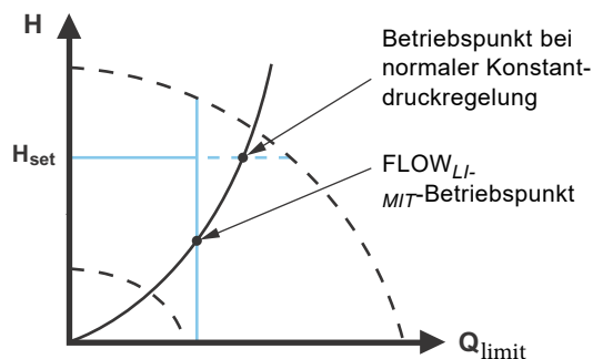
Abb. 40 Konstantdruckregelung mit FLOW LIMIT
