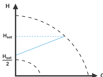
Abb. 28 Proportionaldruckregelung
