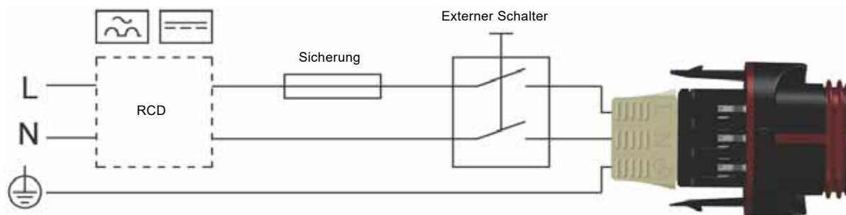
Abb. 11 Beispiel für den Anschluss der Steckerausführung an das Versorgungsnetz mit Hauptschalter, Vorsicherung und FI-Schutzschalter
