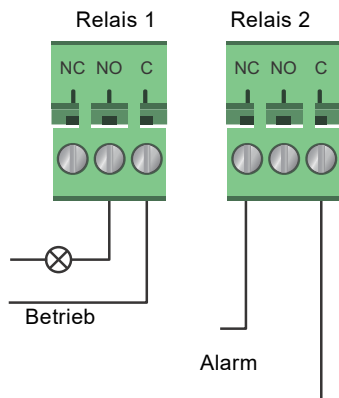
Abb. 46 Relaisausgang
