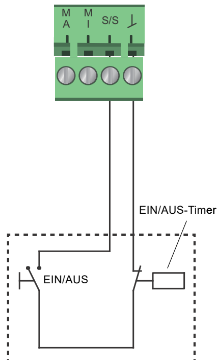
Abb. 47 Digitaleingang
